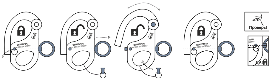
Рис. 3. Открытие / закрытие / фиксация самофиксирующегося запорного элемента.
