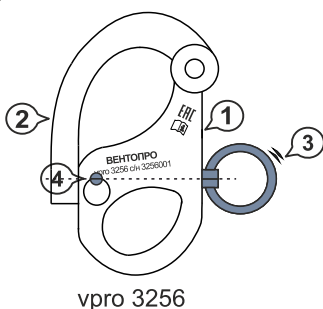
Рис. 2. Маркировка изделий
