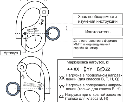
Рис. 2. Маркировка изделий
