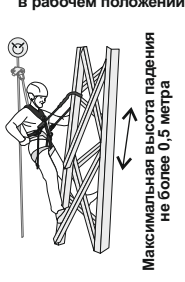
Рис. 12а. Позиционирование в рабочем положении
