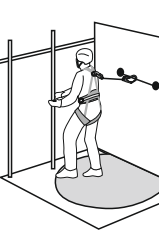
Рис. 11. Способ организации удерживающей системы
