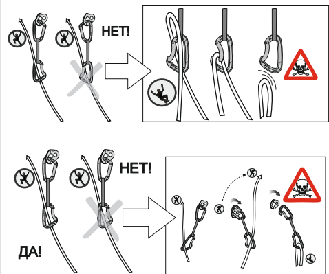
Рис. 3. Прошелкивание веревки
