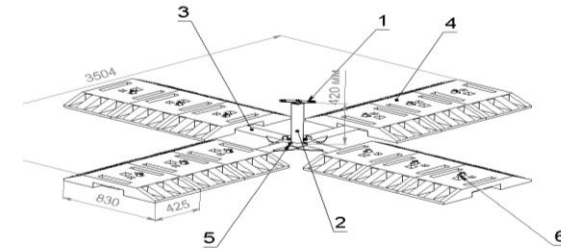
Рис. 1 «Общий вид анкерного устройства «КРЕСТ»: 1. Анкерная точка крепления; 2. Центральный пост-столбик.; 3. Опорная лапа; 4. Противовес; 5. Болт стяжной M12; 6. Штифт предохранительный.
