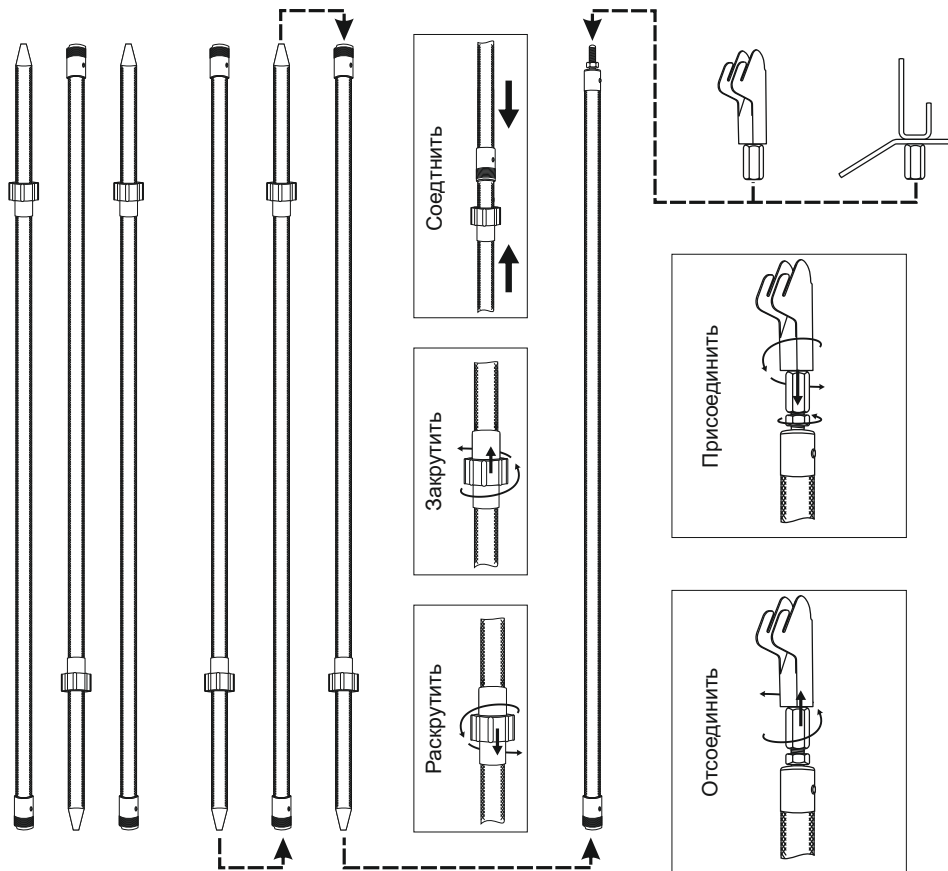
Рис. 2. Сборка
