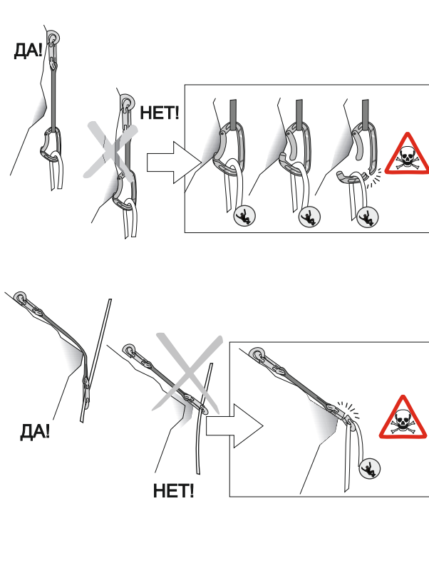
Рис. 4. Установка оттяжек
