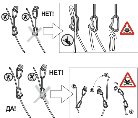
Рис. 3. Прошелкивание веревки
