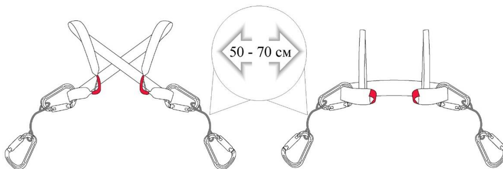
Рисунок 3. Подключение страховочной верёвки и верёвки сопровождения при выполнении ТП по п.п. 7.1, 7.2
